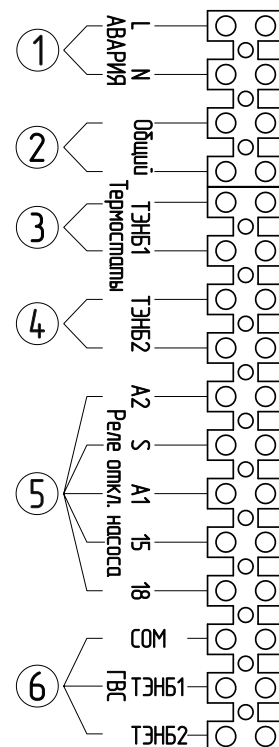
Внешние подключения
