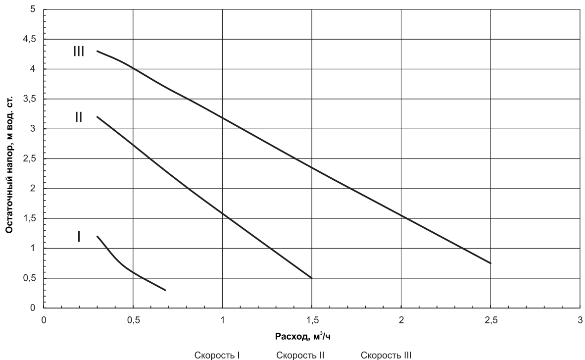
График 1 Остаточный напор для циркуляционного насоса
