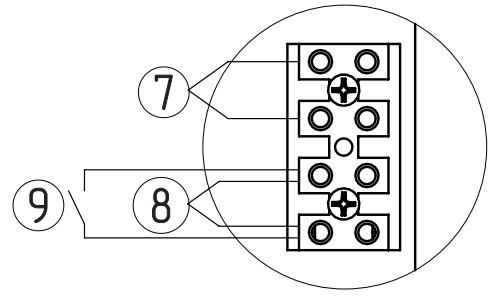
Подключение датчиков
