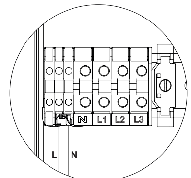
Подключение ИБП или стабилизатора
