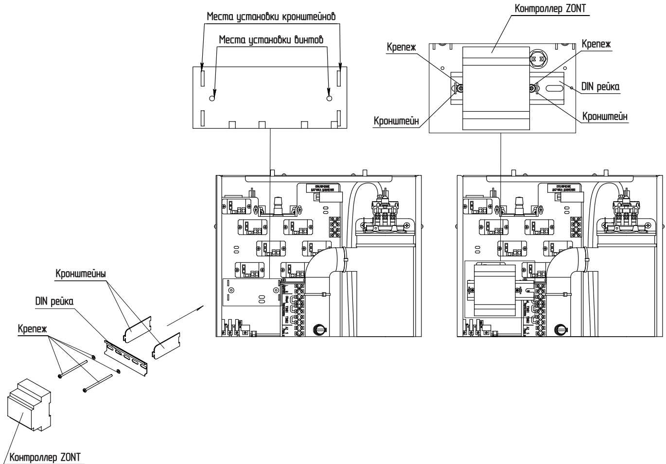
Рис.6 Порядок установки контроллера ZONT для электродкотлов «ТАЕН HEAT»
