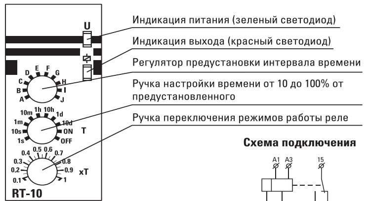
Панель управления
