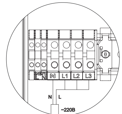
Подключение 220 В
