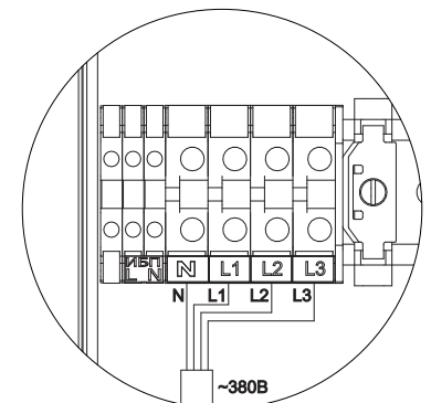
Подключение 380 В
