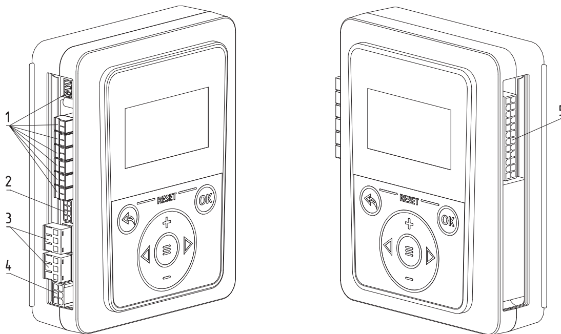
Рис.1 Корпус контроллера «ZOTA X-Line 100E»
