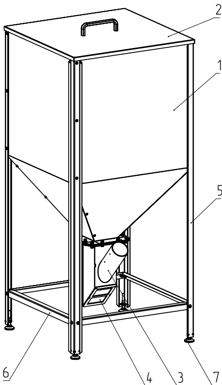
Рис.4. Топливный бункер.
