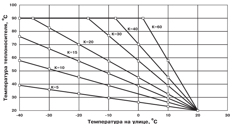
Рис.9 График погодозависимого регулирования
