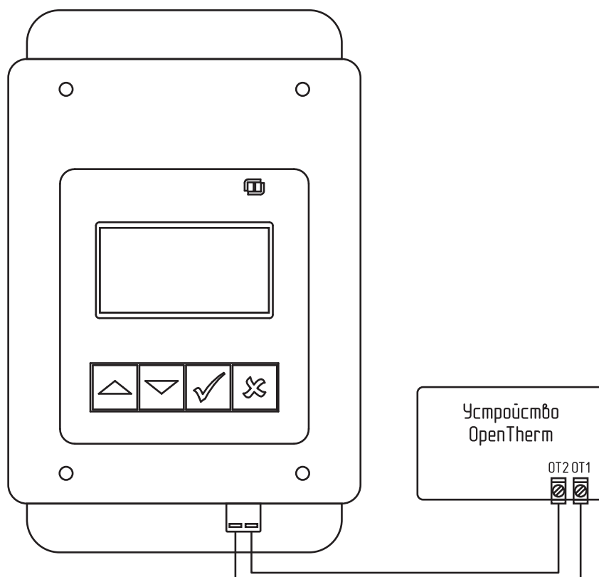
Рис.7 Схема подключения OpenTherm
