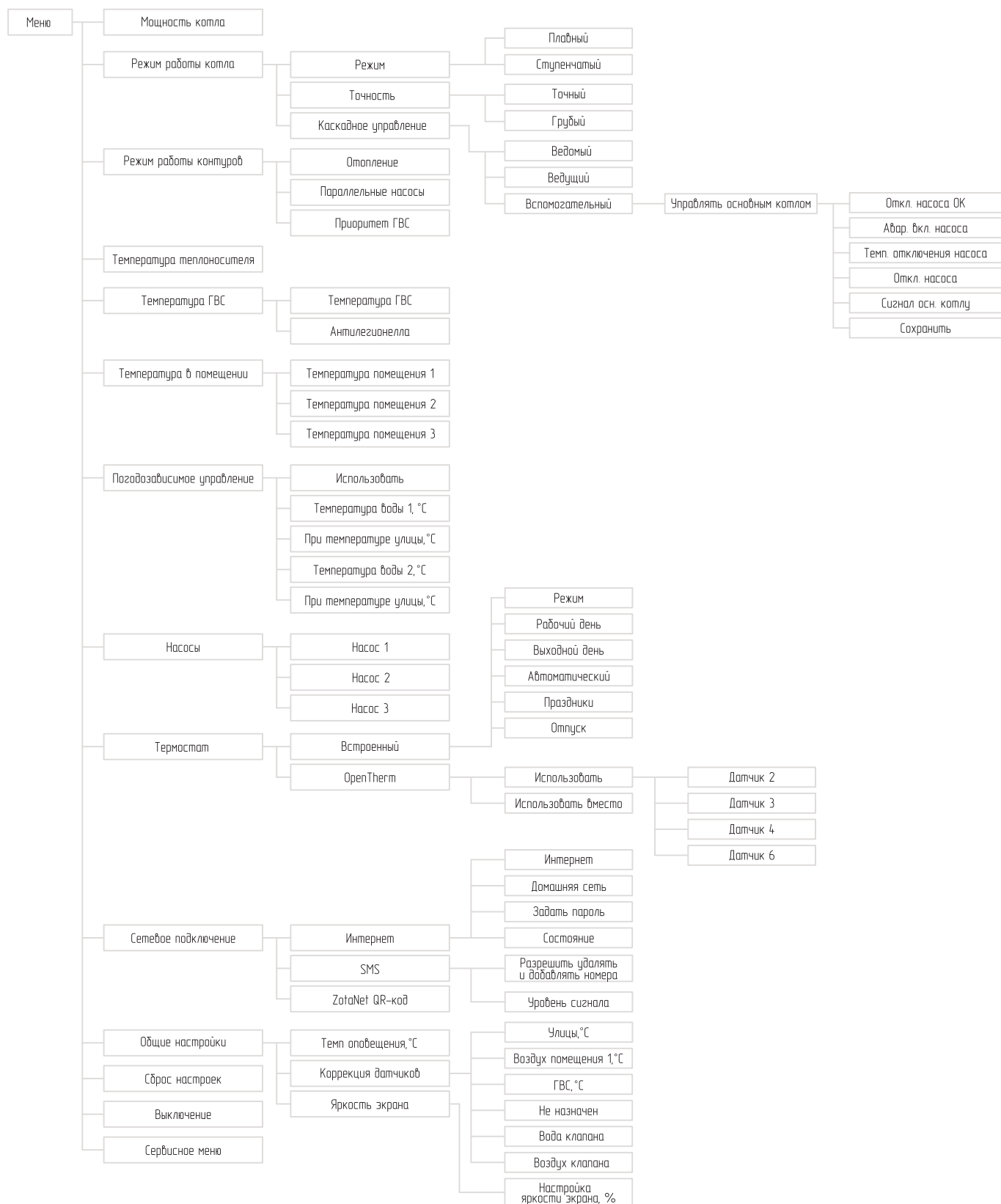
Рис.6 Схема меню пользователя
