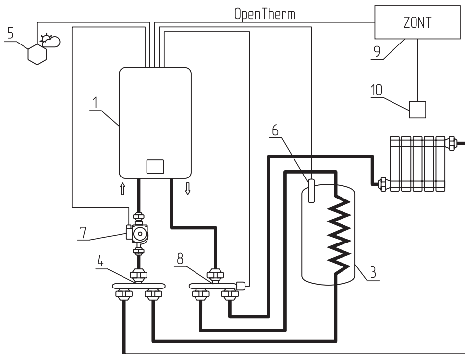
Схема 2. Контур отопления 1 с ГВС, управляемые с помощью переключающего клапана ZONT
