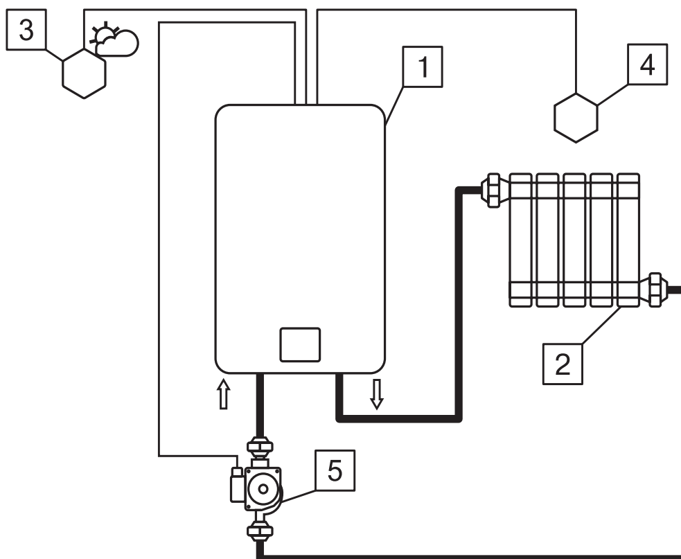
Схема 1. Контур отопления 1 с погодозависимым управлением
