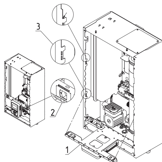
Рис.13 Откидывание кронштейна
