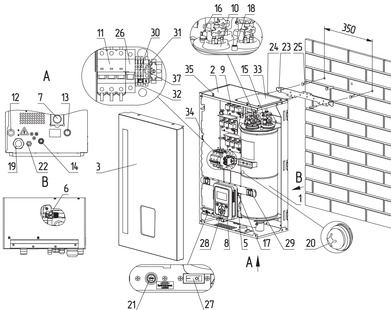
Рис.5 Устройство электрического котла ZOTA MK-X 30-36 кВт
