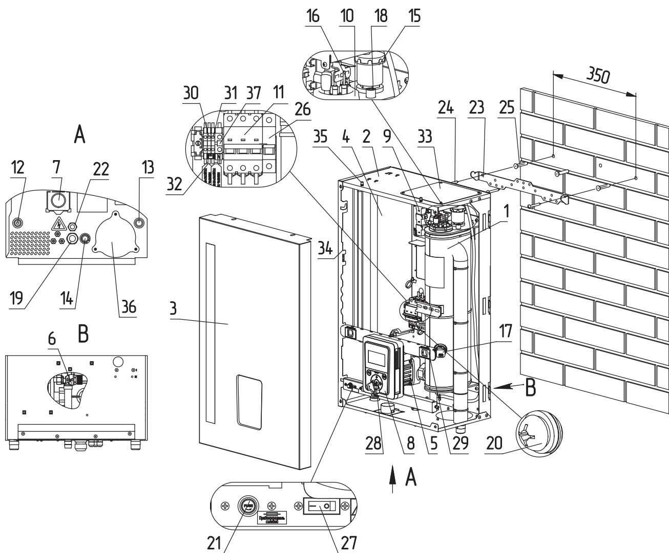
Рис.4 Устройство электрического котла ZOTA MK-X 4,5-24 кВт
