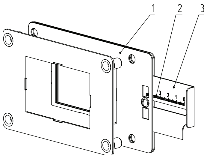
Рис.14 Заслонка вентилятора
